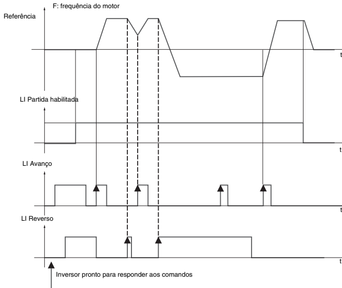
Diagrama de controle a 3 fios (consultar a página 50)
